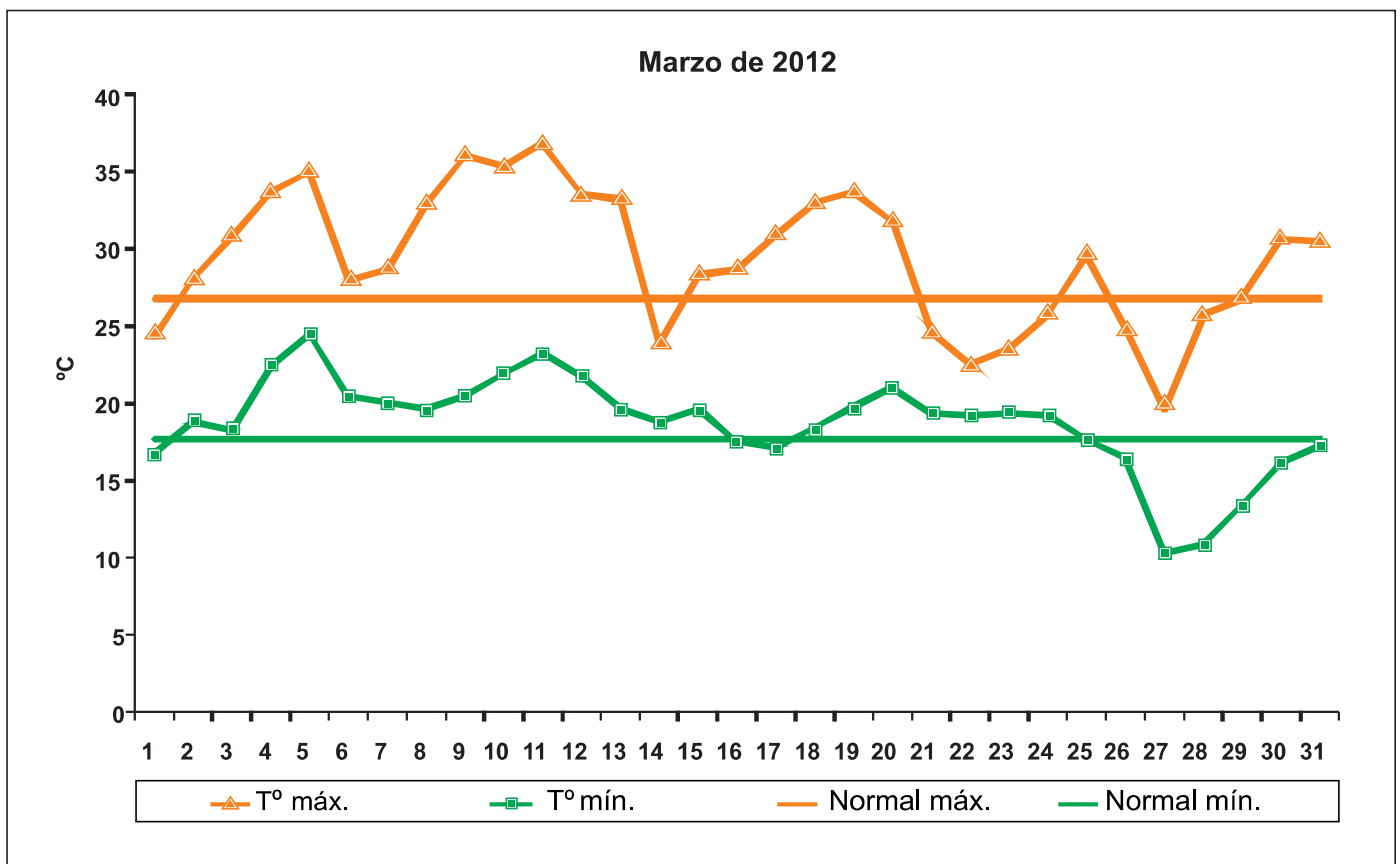
Figura 6. Temperaturas extremas diarias para el mes de marzo de 2012 en la localidad de El Colmenar.
